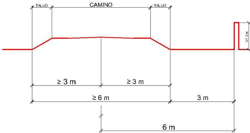
Fig: Protección de los caminos.
