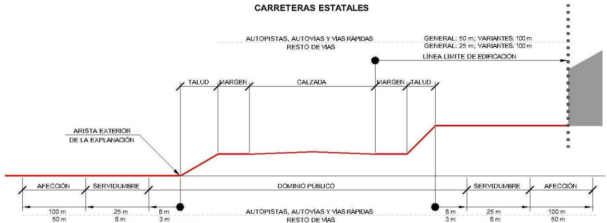
Fig: Protección de carreteras estatales (esquema orientativo)
