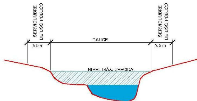
Fig: Protección de desagües naturales
